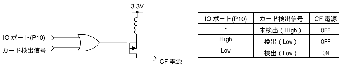
Fig 3.10-3 CF カード電源制御回路
