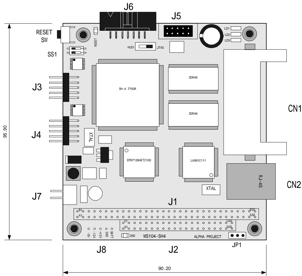
Fig 2.3-1 MS104-SH4 外形図
