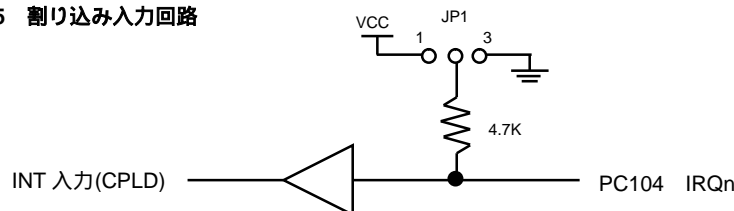
Fig 3.13-5 割り込み入力回路
