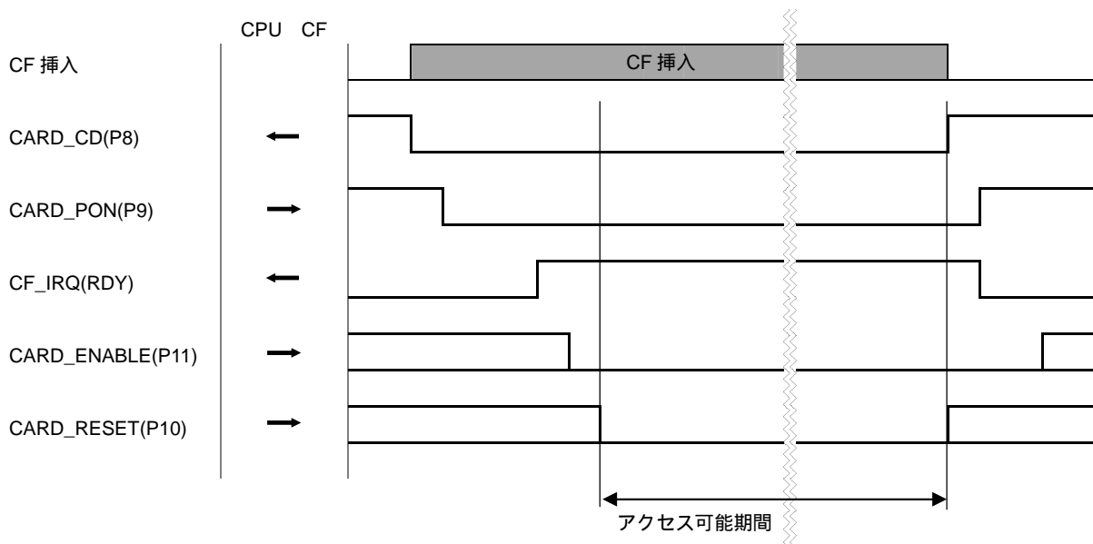
Fig 3.10-5 CF カード初期化タイミング
