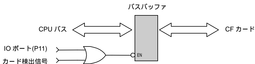
Fig 3.10-4 CF カードインターフェース活性化回路
