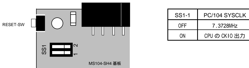
Fig 3.13-4 SS1 の位置
