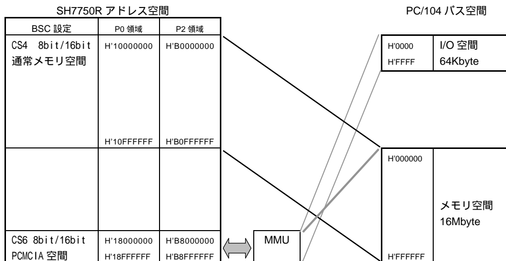
Fig3.13-3 PC/104 バスのマッピング
