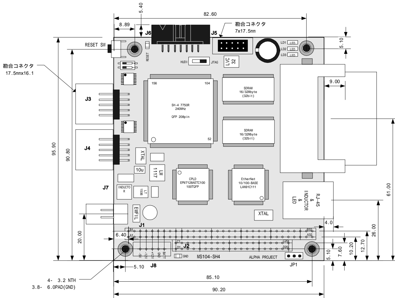
Fig 4.1-1 基板寸法図
