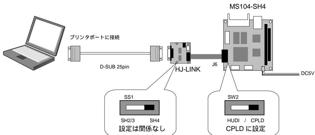
Fig 4.3-1 HJ-LINK の接続
