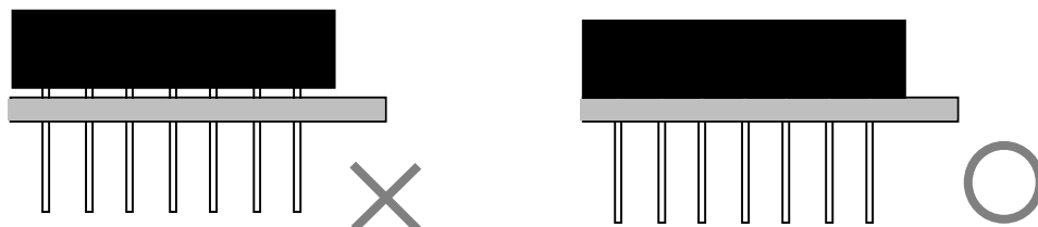
Fig 4.4-1 PC/104 コネクタの実装
