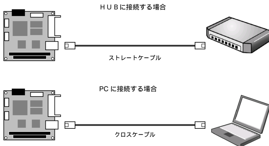
Fig 3.9-2 LAN 接続図
