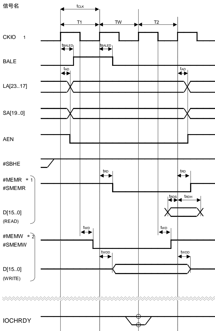
Fig 3.13-8 PC/104 バス SH アクセスタイミング
