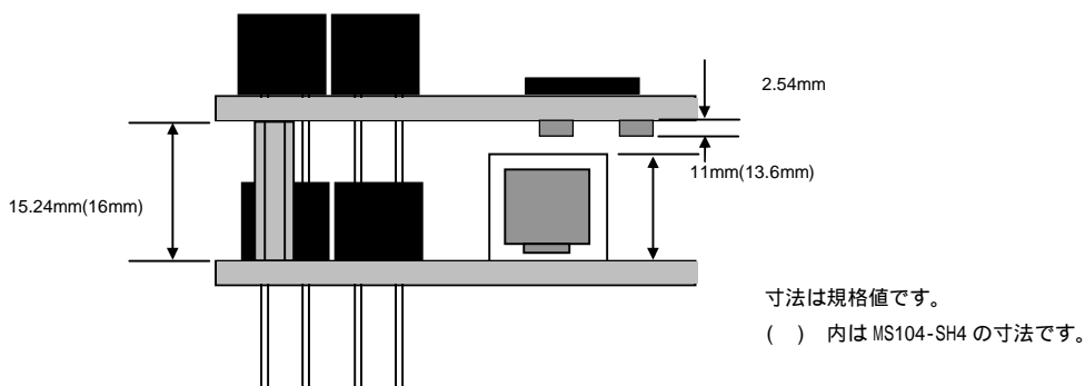
Fig 4.4-2 PC/104 スタッキング寸法図
