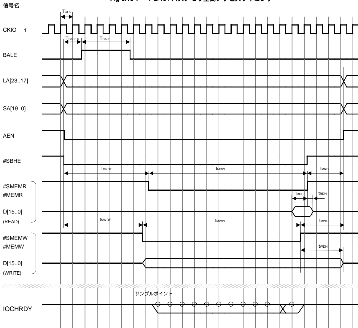
Fig 3.13-7 PC/104 バスメモリ空間アクセスタイミング
