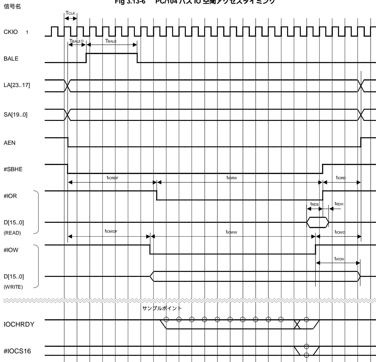
Fig 3.13-6 PC/104 バス IO 空間アクセスタイミング
