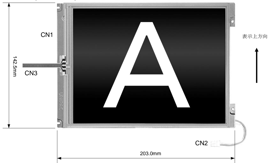
Fig 2.2.1 LCD パネル(97G084S3N1F-2)外形図
