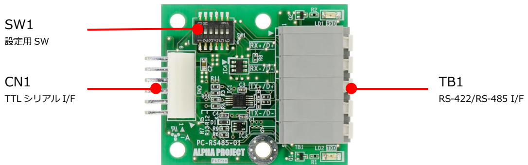
Fig 1.7-1 外形図
