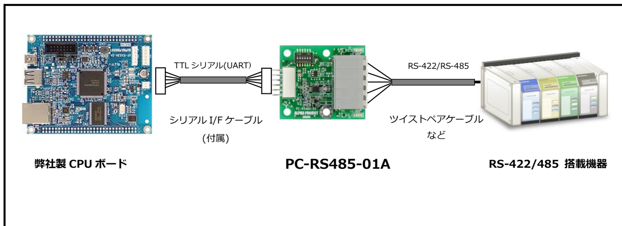
Fig 1.3-1 PC-RS485-01A 接続イメージ
