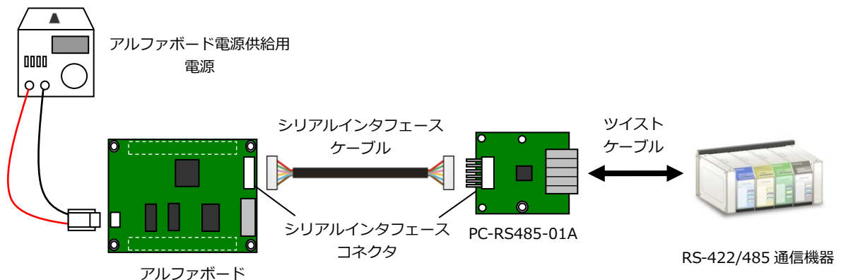
Fig 3.2-1 PC-RS485-01A とアルファボードとの接続例
