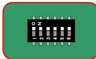
出荷時設定：RS485/2 線式/終端抵抗 ON
