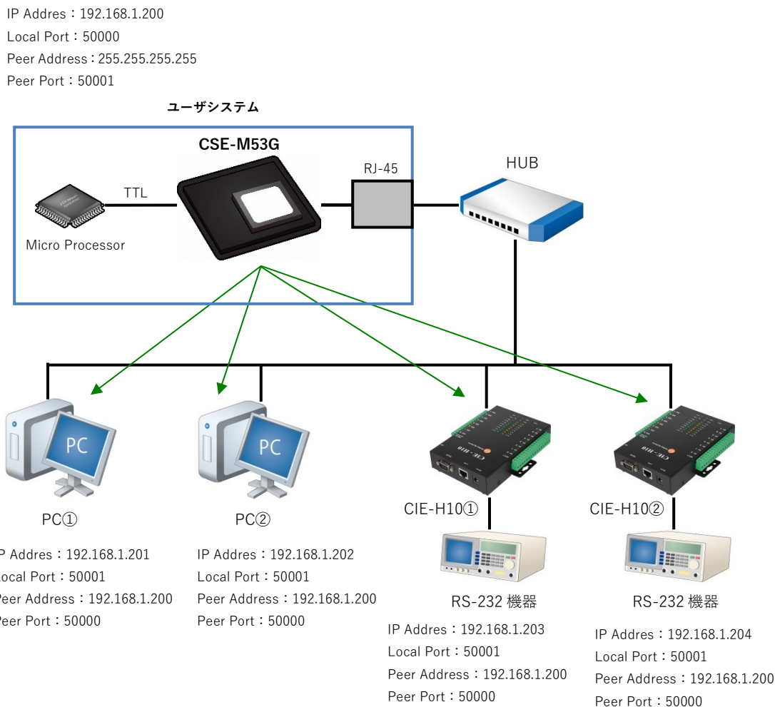
Fig 5.7-5 ブロードキャスト通信構成例
