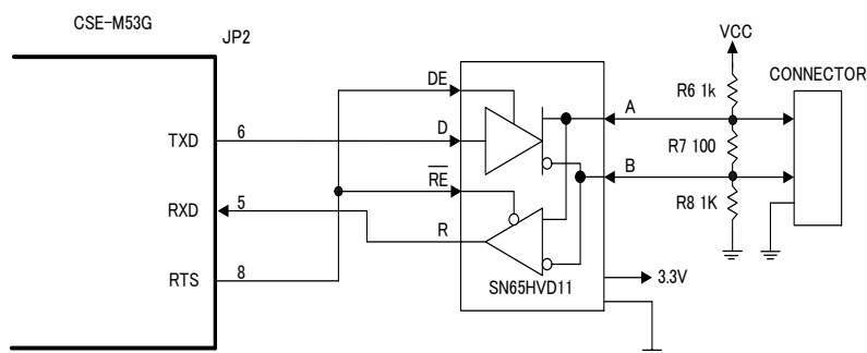
Fig 8.1-5 RS485 ドライバの接続
