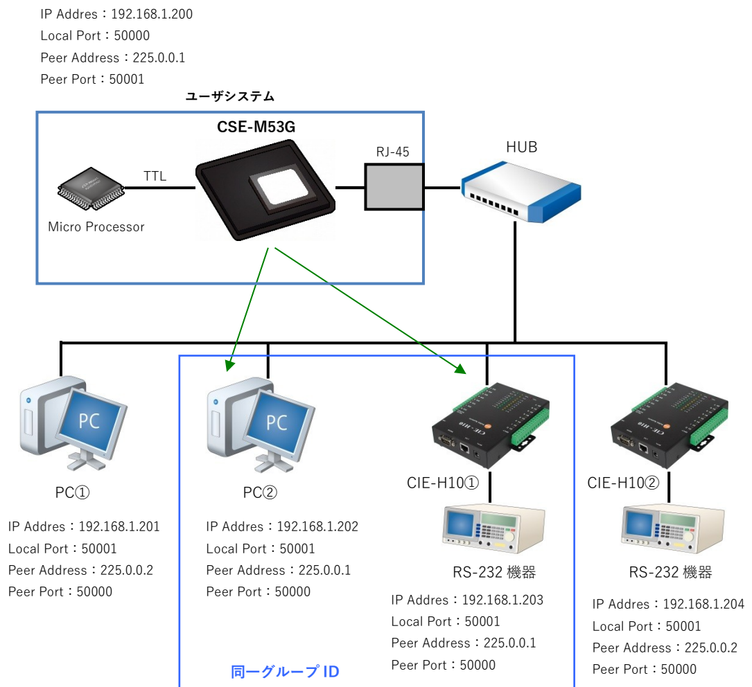
Fig 5.7-6 マルチキャスト通信構成例
