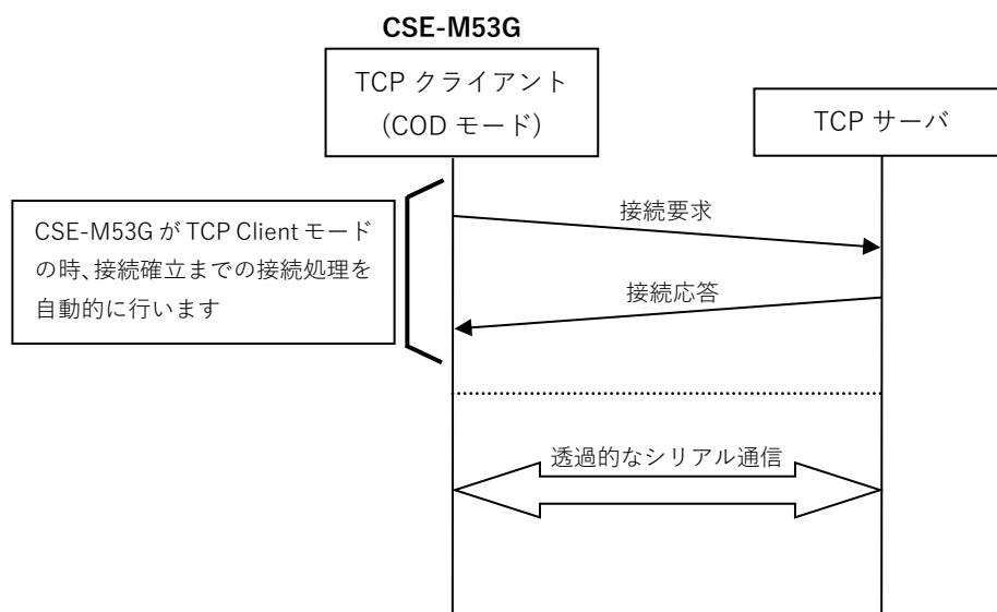
Fig 5.5-1 TCP Client モード接続手順
