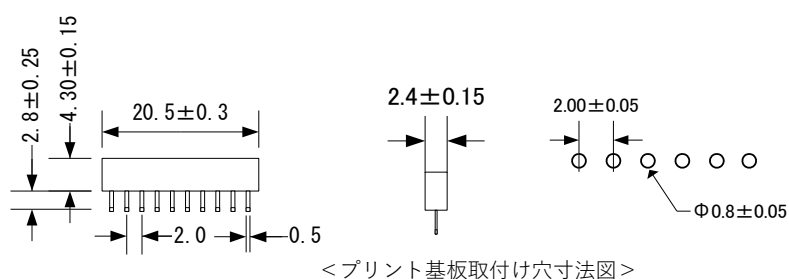
Fig 1.6-2 レセプタクル (付属) (型番 SD1-10:AUK 社)
