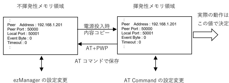
Fig 3.3-2 保存設定値と動作設定値の関係
