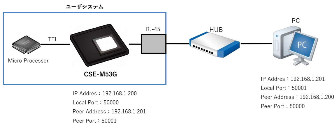
Fig 5.7-3 ユニキャスト通信構成例 1
