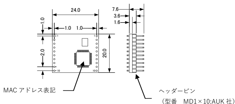
Fig 1.6-1 外形寸法図
