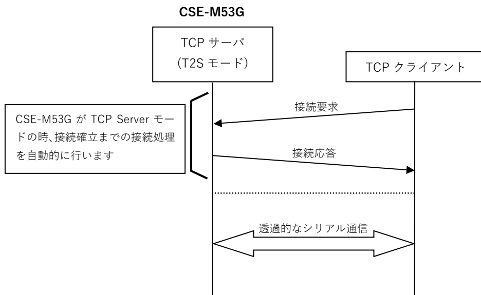
Fig 5.4-1 TCP Server 接続手順
