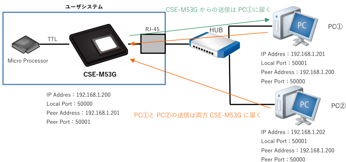
Fig 5.7-4 ユニキャスト通信構成例 2
