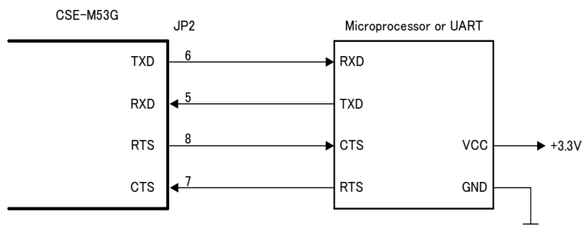
Fig 8.1-2 3.3V マイコンの接続
