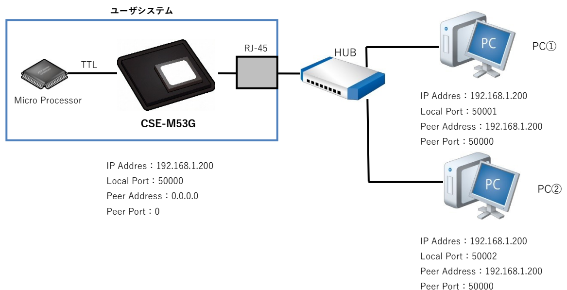
Fig 5.7-7 U2S エコー通信構成例
