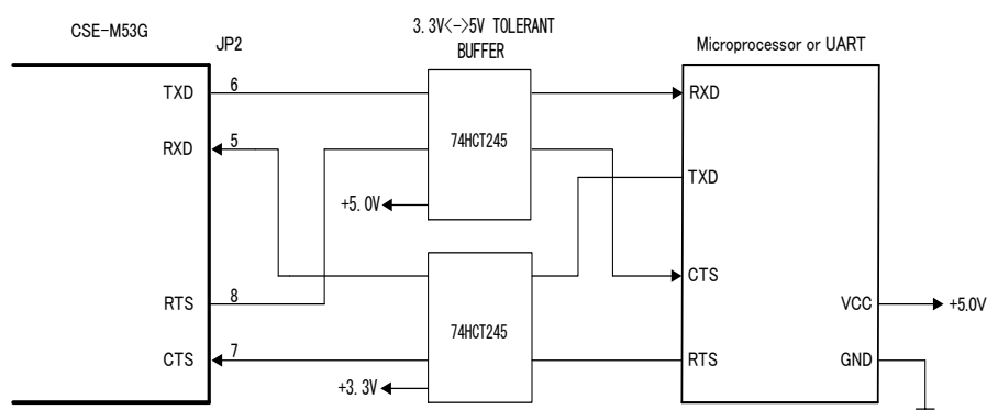
Fig 8.1-3 5.0V マイコンの接続
