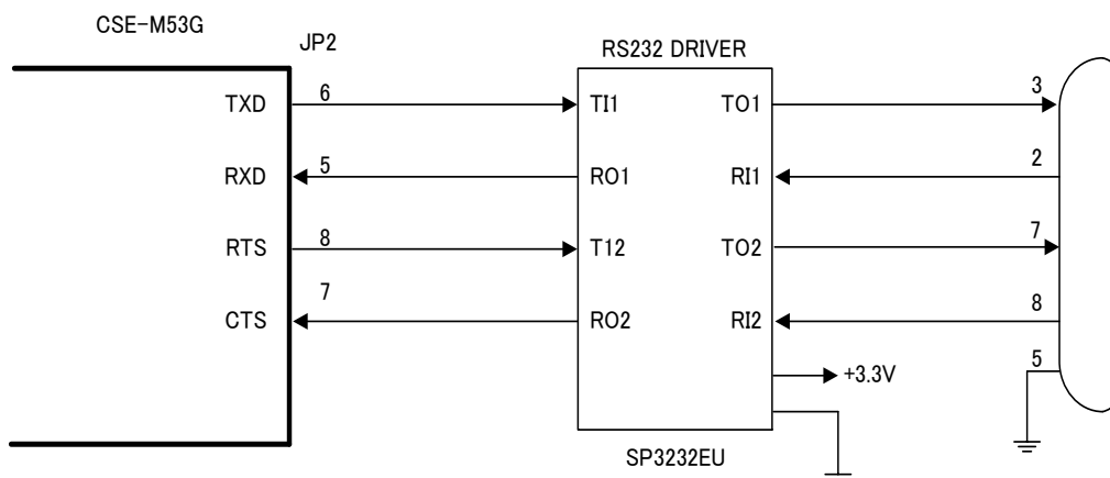
Fig 8.1-4 RS232 ドライバの接続
