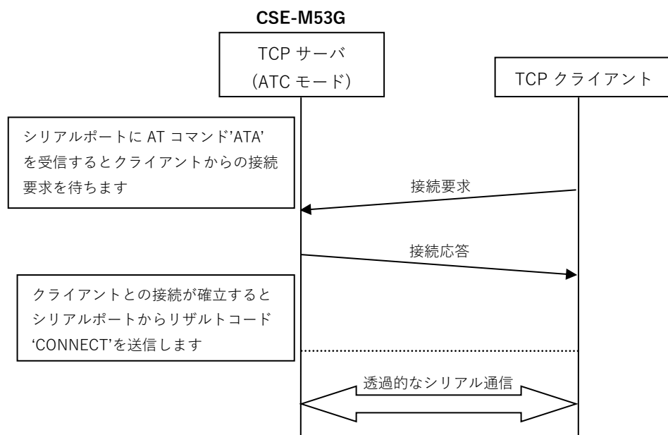
Fig 5.6-1 AT Command モード接続手順 (TCP クライアントとの接続)
