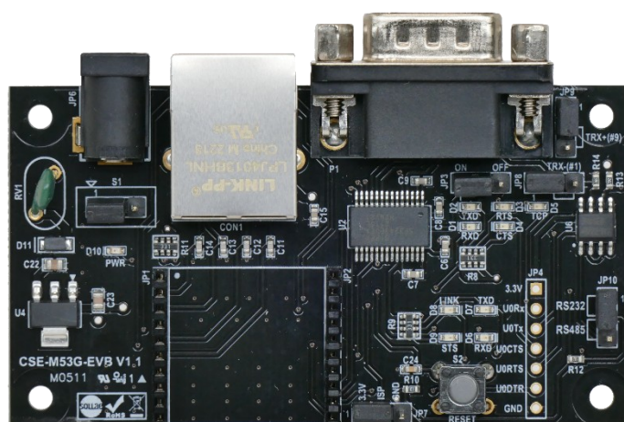
CSE-M53G EVA ボード
