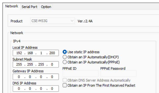
Fig 5.2-2 ezManager IPv4 設定欄
