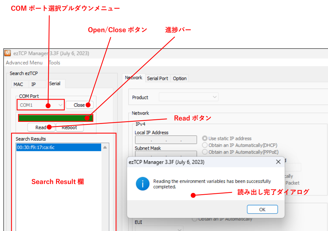
Fig 3.2-8 ezManager シリアルインタフェースからの設定値読み出し
