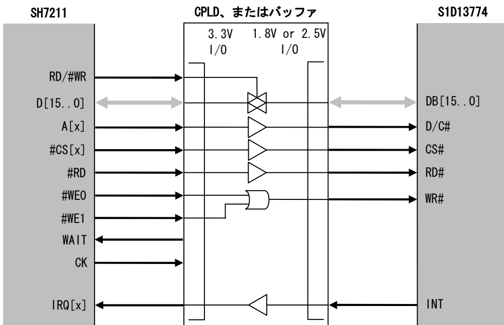
Fig 2.2-1 接続例
