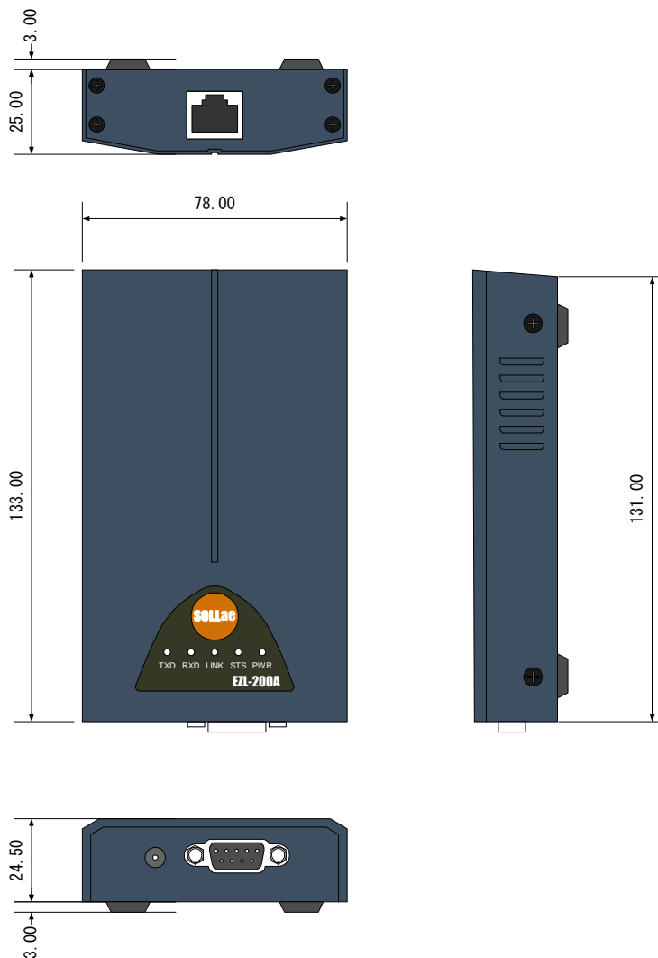
図2. 1-1 外形寸法図
