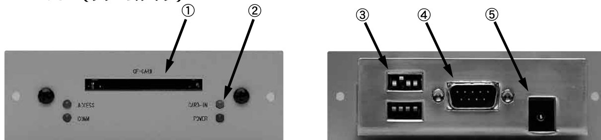
①CFカードスロット ②表示LED ③動作設定用DIP-SW ④9ピンDサブコネクタ (EIA-574) ⑤ACアダプタジャック
