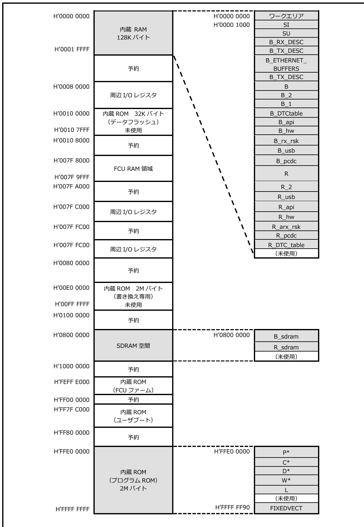
Fig 3.2-1 ネットワーク通信 + USB ファンクションサンプルプログラムメモリマップ
